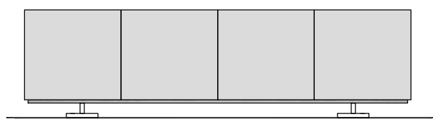
1600-4D ( deuren ) incl. onderstel 1600-4K ( + klep ) incl. onderstel 1600-4L ( + lade ) incl. onderstel 1840 x 510 x 500
