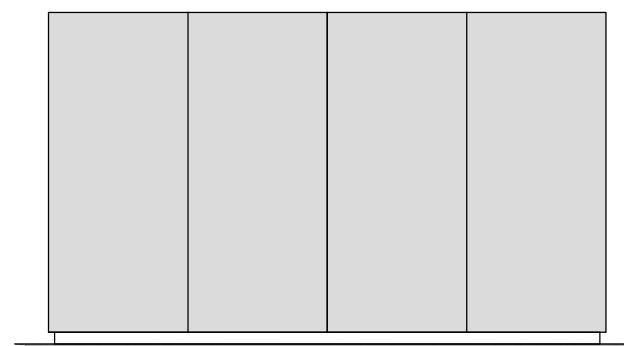
820L + 820R 1600.840 ( 4 deuren ) incl. plint 1840 x 1092 x 500
