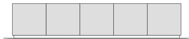
1600-5D ( deuren ) incl. plint 1600-5K ( + klep ) incl. plint 1600-5L ( + lade ) incl. plint 2300 x 470 x 500
