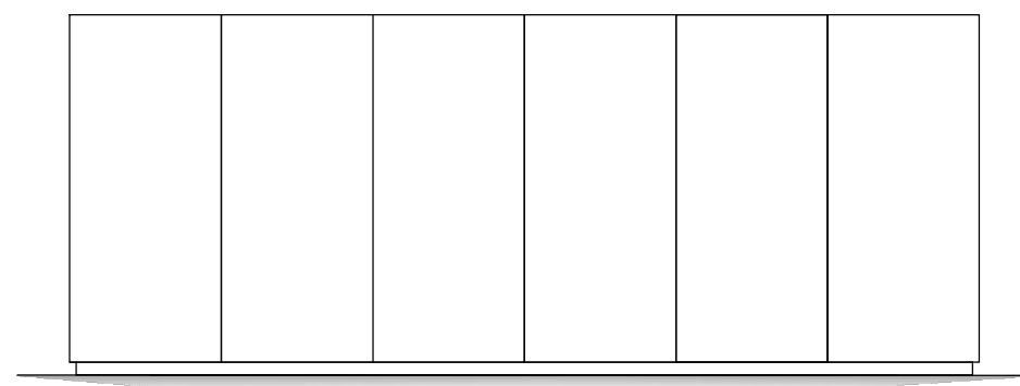
820L + 820M + 820R 1600.860 ( 6 deuren ) incl. plint 2760 x 1092 x 500
