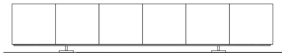
1600-6D ( deuren ) incl. onderstel 1600-6K ( + klep ) incl. onderstel 1600-6L ( + lade ) incl. onderstel 2760 x 510 x 500
