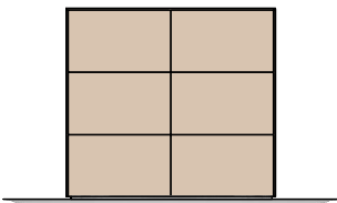
1500.940 (= 920+920) 1384 x 1290 x 444
